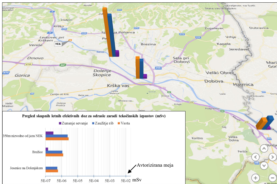
Slika P2: Pregled ocenjenih letnih efektivnih doz za umetne radionuklide za tekočinske izpuste iz NEK v letu 2020
