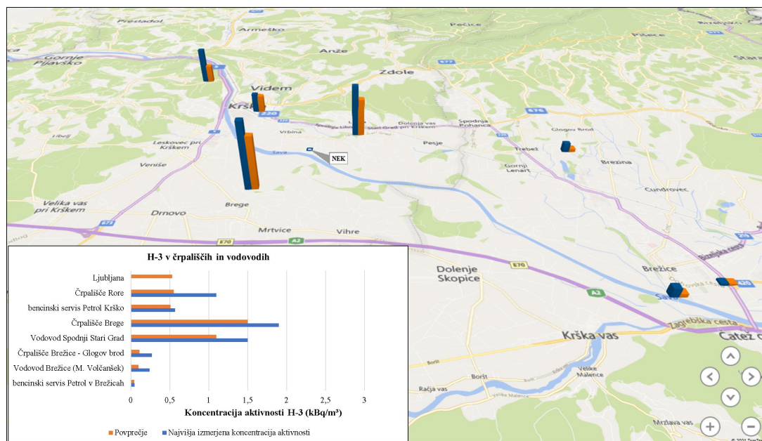
Slika I5: Pregled povprečnih in najvišjih izmerjenih koncentracij aktivnosti H-3 v pitni vodi iz črpaljšč in vodovodov v krški in brežiški občini. na lokacijah, kjer se vzorčujejo neprekinjeno ali četrtletno.
