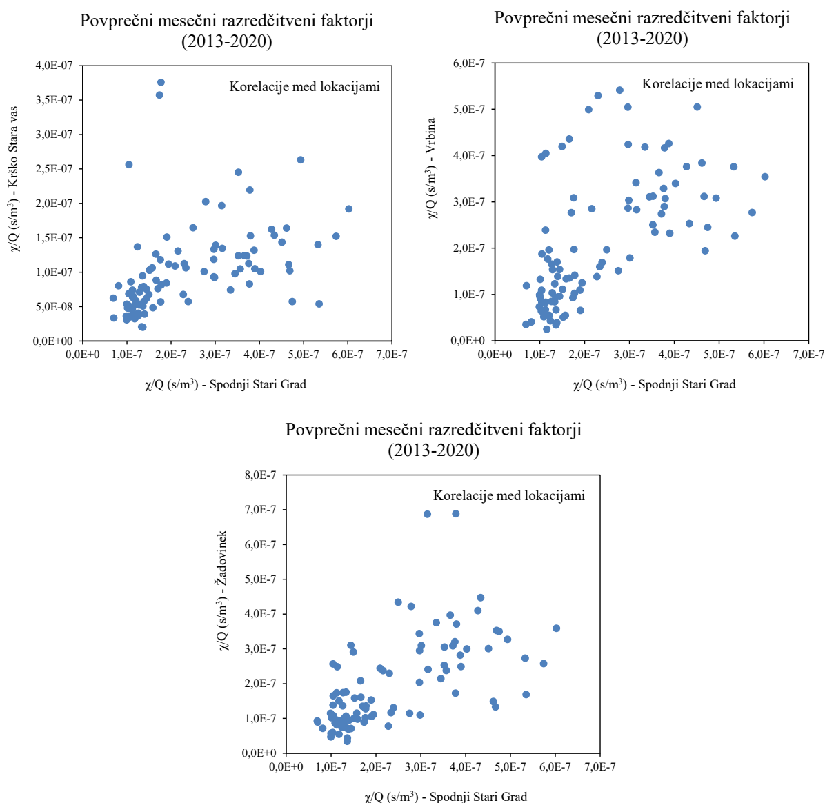
Slika 4.7: Korelacija povprečnih mesečnih razredčitvenih koeficientov ( \chi/Q ) z enoto s/m 3 , na referenčni lokaciji Spodnji Stari Grad in v bližnjih naseljih za leta 2013–2020.
