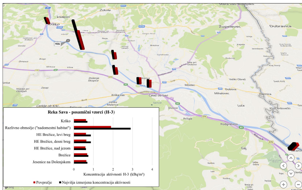
Slika I2: Pregled povprečnih in najvišjih izmerjenih koncentracij aktivnosti H-3 v reki Savi na lokacijah vzvodno in nizvodno od jezua NEK, kjer se vzorčujejo posamični (mesečni ali četrtletni) vzorci.
