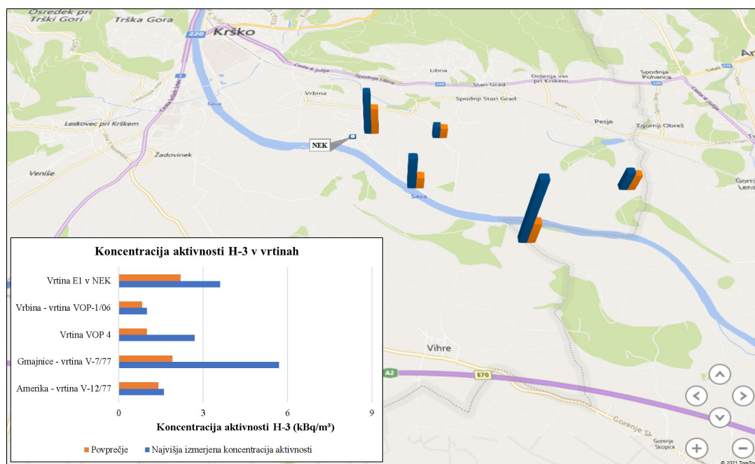
Slika I6: Pregled povprečnih in najvišjih izmerjenih koncentracij aktivnosti H-3 v vodi iz vrtin.
