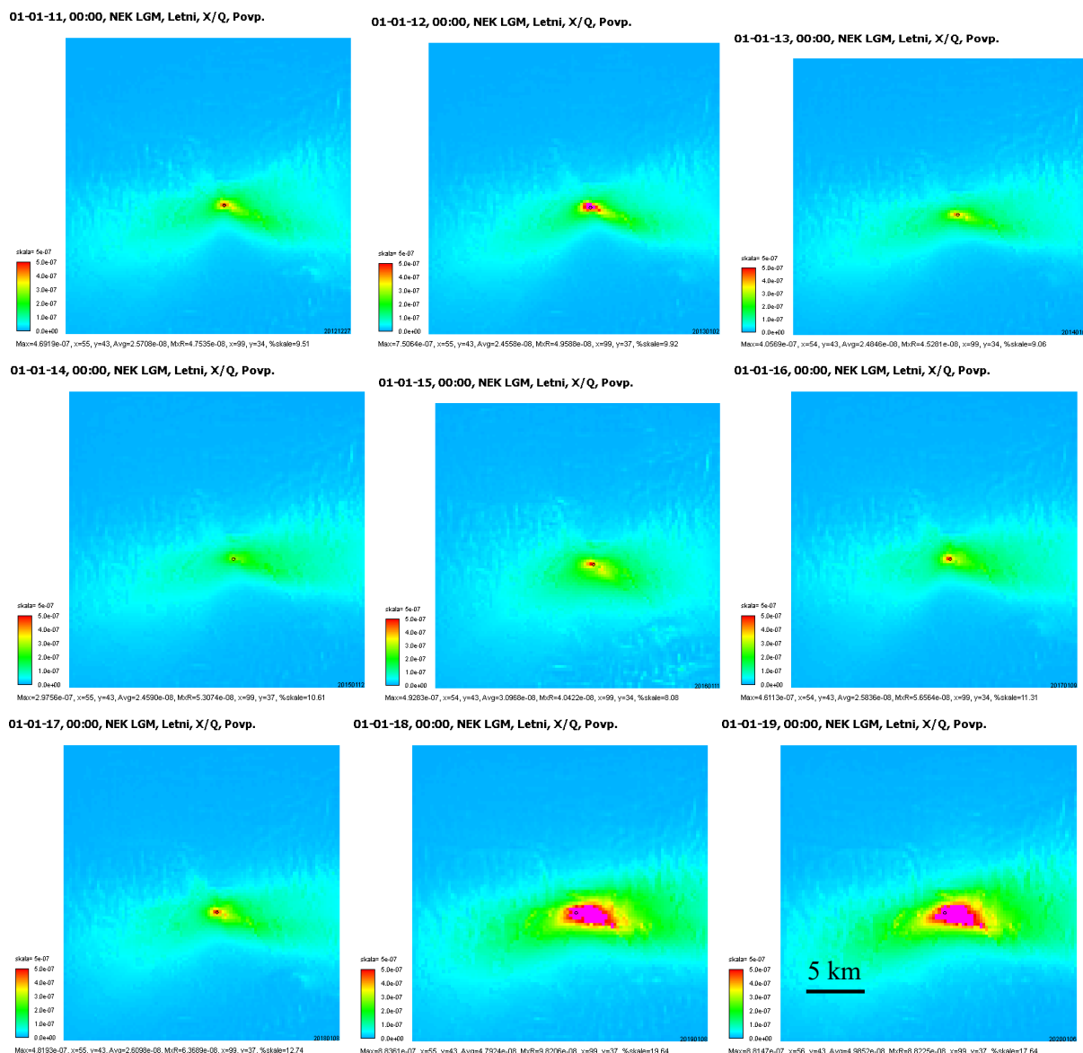
Slika 4.5b: Povprečni letni razredčitveni koeficienti ( \chi/Q ) z enoto \text{s/m}^3 , izračunani po Lagrangeevem modelu za izpust z višine 60 m za okolico NEK za leta 2011–2019 Podatke je izračunal in posredoval MEIS storitve za okolje
