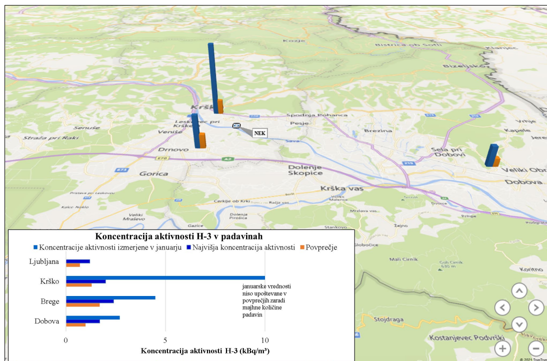
Slika I7: Pregled povprečnih in najvišjih izmerjenih koncentracij aktivnosti H-3 v padavinah
