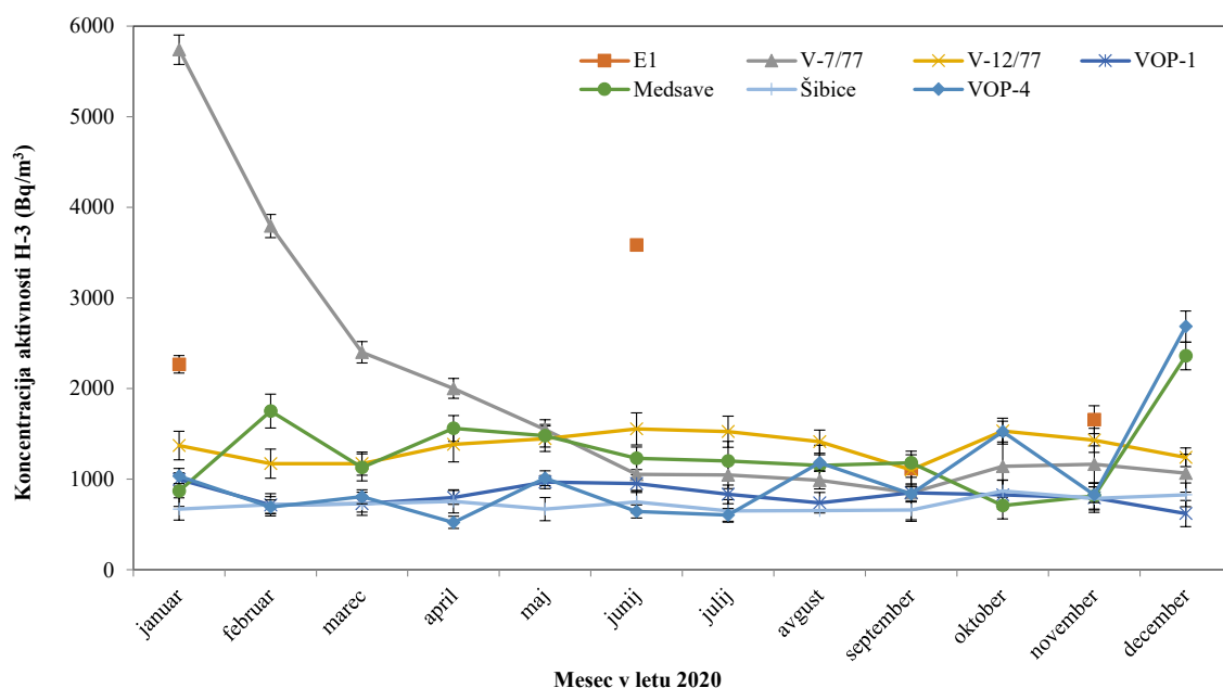
Slika 2.2: Koncentracija aktivnosti H-3 v mesečnih vzorcih vrtin.
