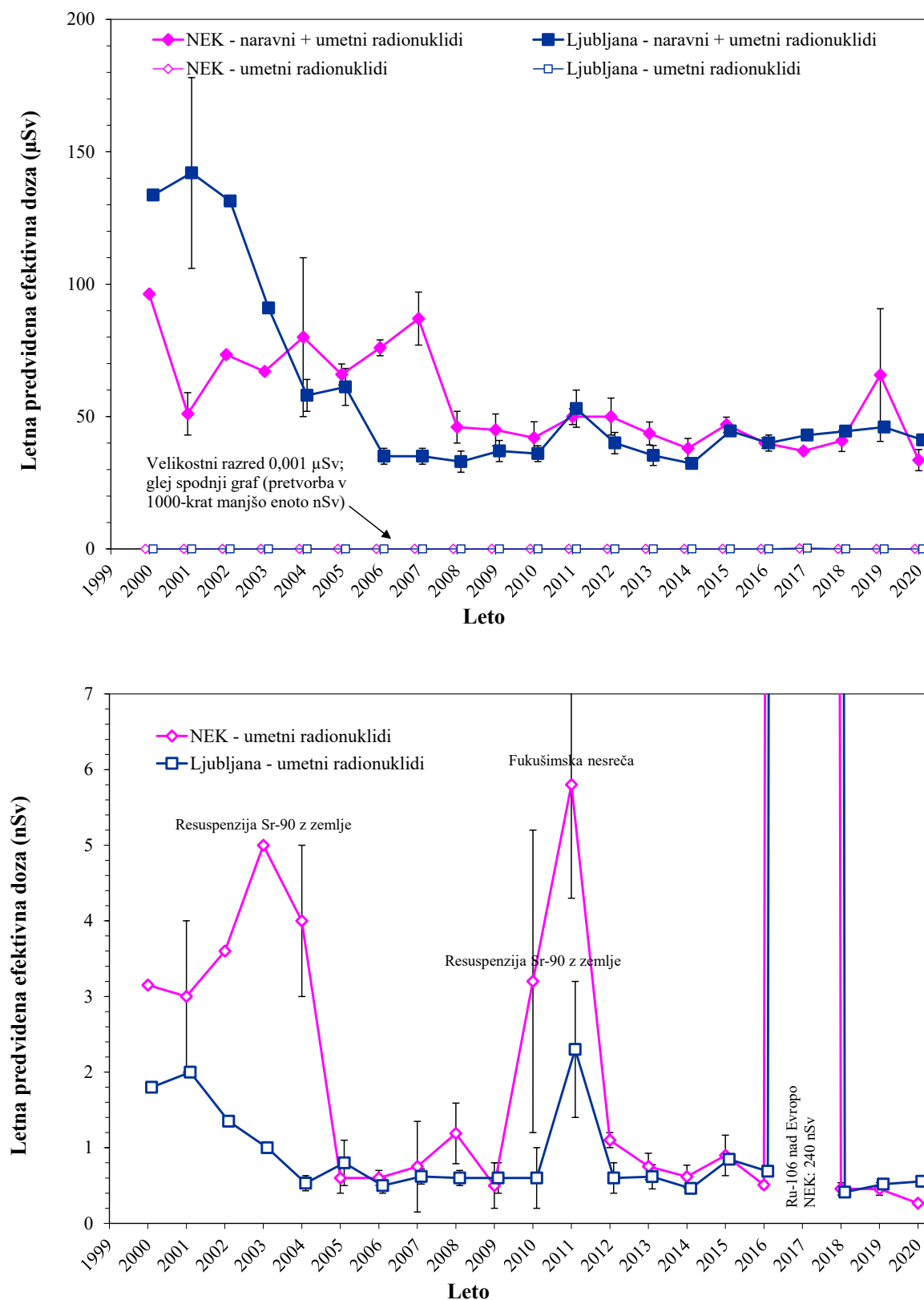
Slika 4.8: Primerjava letnih predvidenih efektivnih okoljskih doz za leto 2020 v okolici NEK in Ljubljani za odrasle osebe iz meritev aerosolov za naravne in umetne radionuklide skupaj v enotah \mu\text{Sv} (zgornja slika) in posebej za umetne radionuklide v 1000-krat manjši enoti nSv (spodnja slika). Vrisane negotovosti imajo faktor pokritja k = 1 (68-odstotna zanesljivost).
