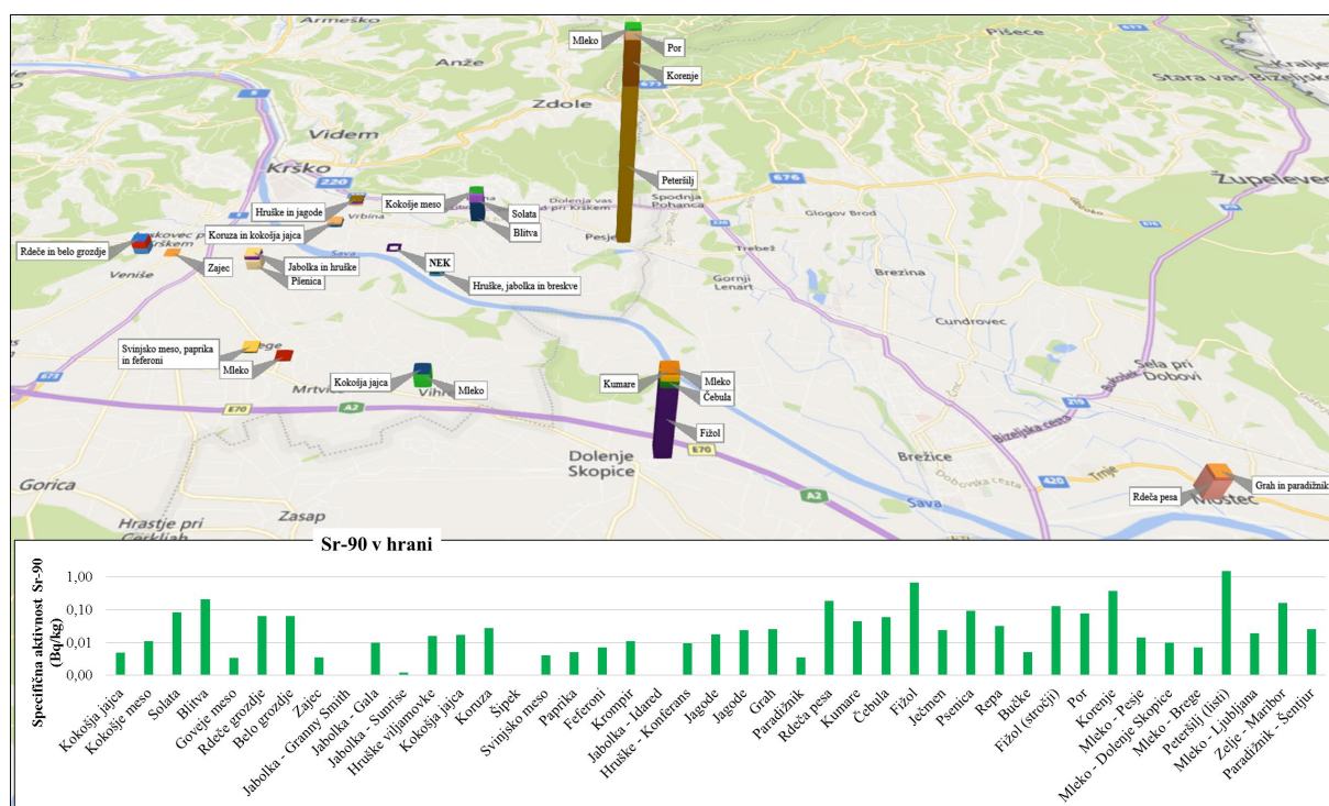
Slika I14: Specifične aktivnosti Sr-90 v hrani v okolici NEK v letu 2020
