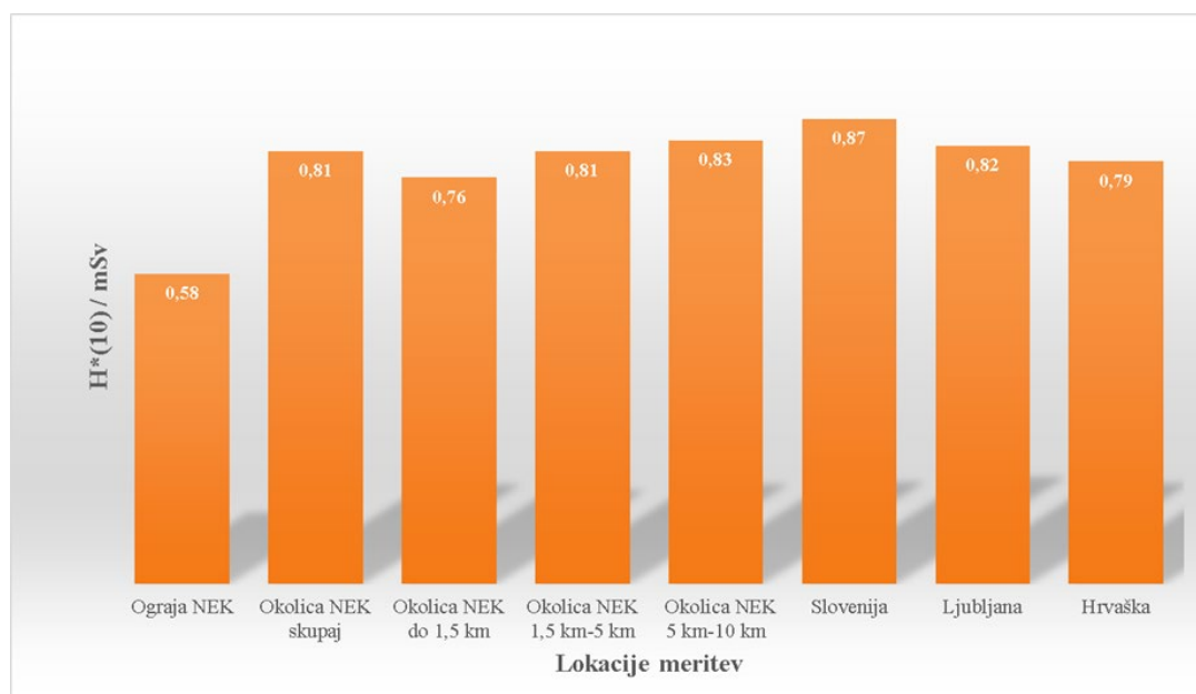
Slika I9: Primerjava med povprečnimi okoljskimi doznimi ekvivalenti H^*(10) , izmerjenimi v okolici NEK, na referenčni lokaciji v Ljubljani in povprečnimi ekvivalenti izmerjenimi na Hrvaškem v okviru programa nadzora radioaktivnosti v okolici NEK ter povprečnimi ekvivalenti izmerjenimi v okviru meritev radioaktivnosti v življenjskem okolju v Republiki Sloveniji.
