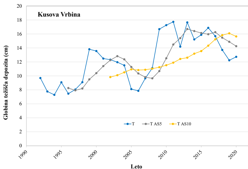
Slika 5.1c: Globina težišča nanosa Cs-137, izračunanega na podlagi letnih vzorčenj za lokacijo Kusova Vrbina. Prikazano je tudi 5-letno (T AS5) in 10-letno (T AS10) drseče povprečje globine težišča depozita.
