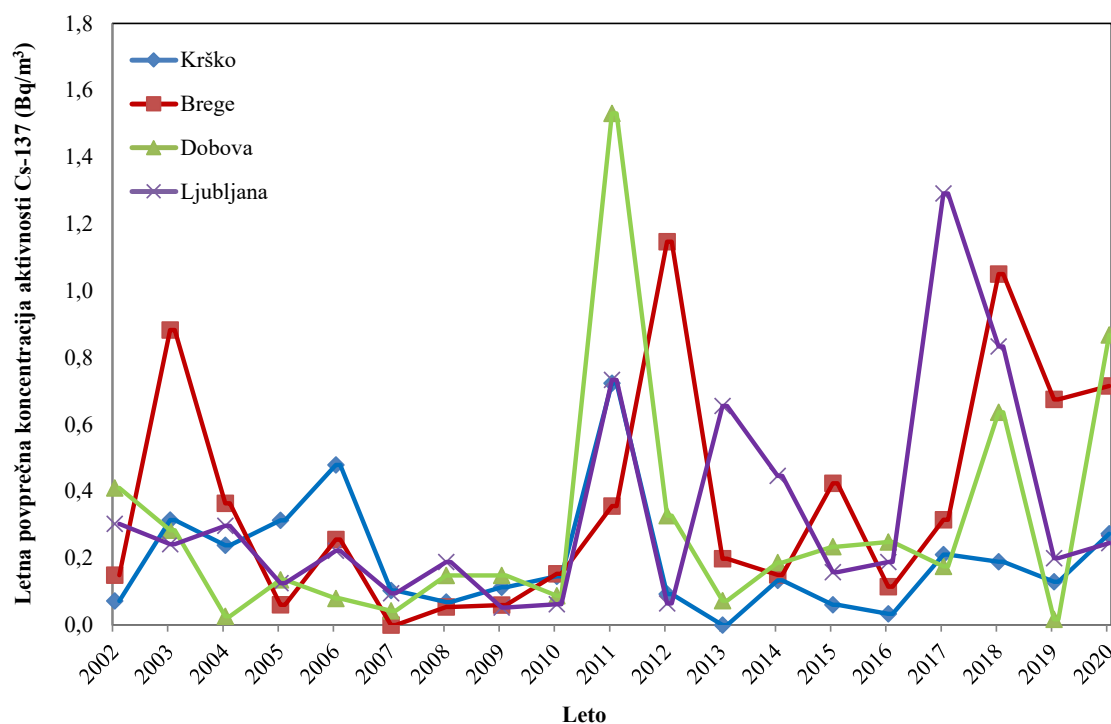
Slika 3.7: Letna koncentracija aktivnosti Cs-137 v padavinah za obdobje 2006–2020. Izrazito povišanje v letu 2011 na vseh vzorčevalnih mestih je posledica nesreče v Fukušimi.
