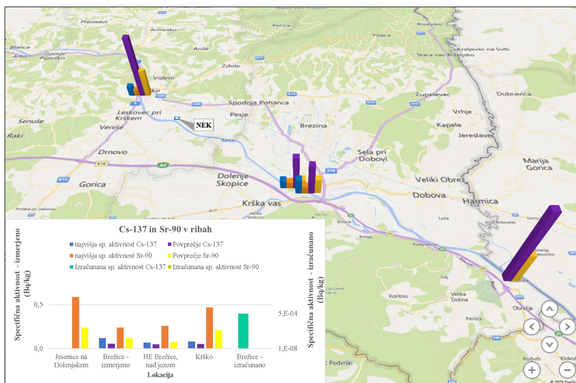
Slika I4: Specifične aktivnosti Cs-137 in Sr-90 v ribah v letu 2020
