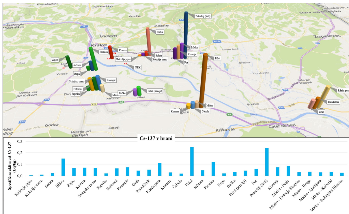
Slika I13: Specifične aktivnosti Cs-137 v hrani v okolici NEK v letu 2020
