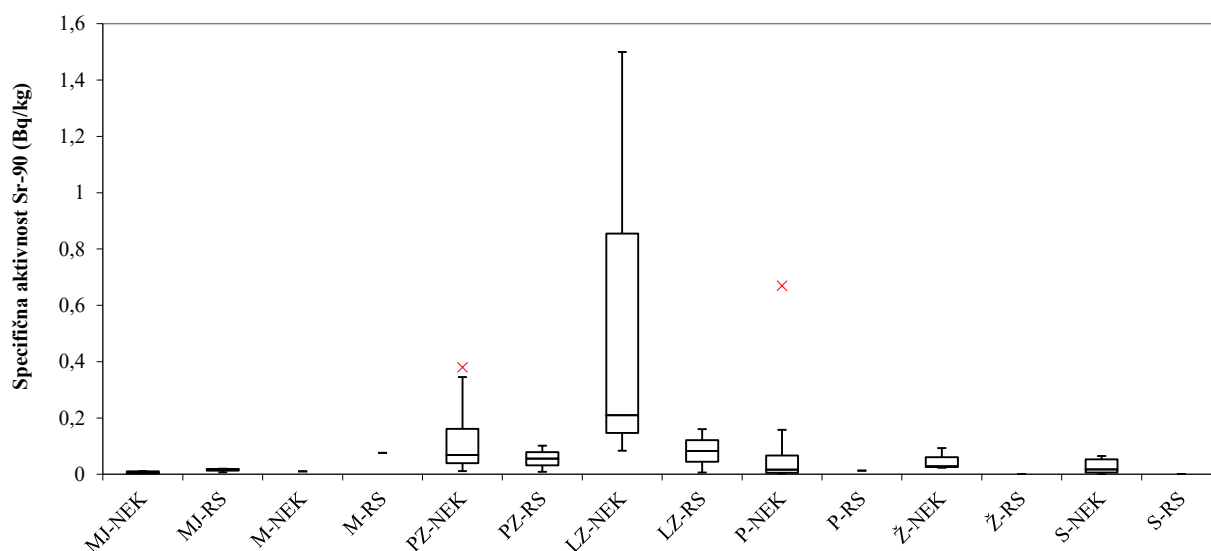
Slika 6.3: Specifična aktivnost Sr-90 (Bq/kg) v skupinah žvil: MJ – meso in jajca, M – mleko, PZ – podzemna zelenjava, LZ – listna zelenjava, P – plodovke, Ž – žita, S – sadje; predstavljene so minimalna in maksimalna vrednost (brki) ter mediana, prvi in tretji kvartil (pravokotnik) po skupinah posamično vzorčenih žvil v letu 2020 v okolici NEK in drugod po Sloveniji (RS). Izjema je surovo mleko, ki se v okviru obratovalnega nadzora radioaktivnosti v okolici NEK zbira in analizira mesečno na treh lokacijah (Vihre, Pesje in Brege), v okviru nadzora radioaktivnosti v življenjskem okolju v RS pa dvomesečno na treh lokacijah (Ljubljana, Kobarid in Bohinjska Bistrica). V grafu so tako prikazane aritmetične sredine čez vse vzorce v okviru nadzora radioaktivnosti za celo leto 2020. V predstavitvi po živilih so bila upoštevana žvila, ki spadajo v izbrano skupino; nabor žvil v okviru Monitoringa radioaktivnosti v življenjskem okolju v RS obsega še druge vrste žvil, kot so med, ribe, moka itd., ki se v okviru obratovalnega nadzora radioaktivnosti v okolici NEK ne vzorčujejo. Če je bilo odvzetih več vzorcev iste vrste, je v tabeli poročana aritmetična sredina. Z znakom – so označene posamične meritve, z znakom × pa ubežniki (angl. outliers ).
