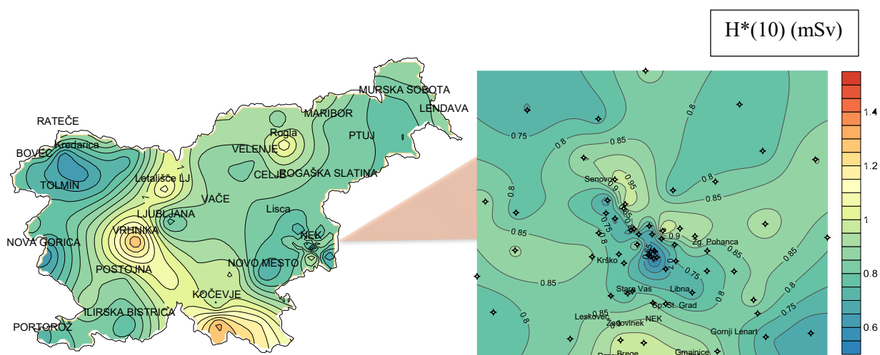
Slika I10: Povprečni letni okoljski dozni ekvivalent H^*(10) po Sloveniji in v okolici NEK v letu 2020
