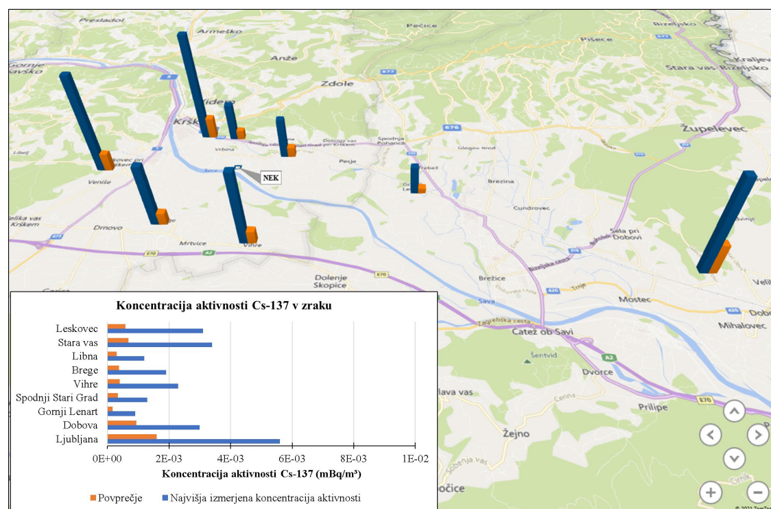
Slika I8: Pregled povprečnih in najvišjih izmerjenih koncentracij aktivnosti Cs-137 v zraku
