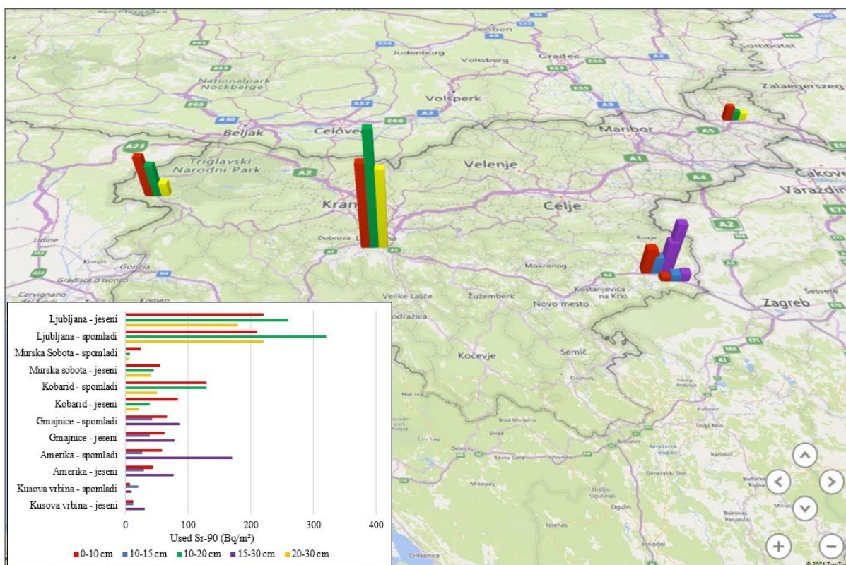
Slika I12: Usedi Sr-90 po Sloveniji (Ljubljana, Murska Sobota, Kobarid) in v okolici NEK (Gmajnice, Amerika, Kusova Vrbina) v letu 2020
