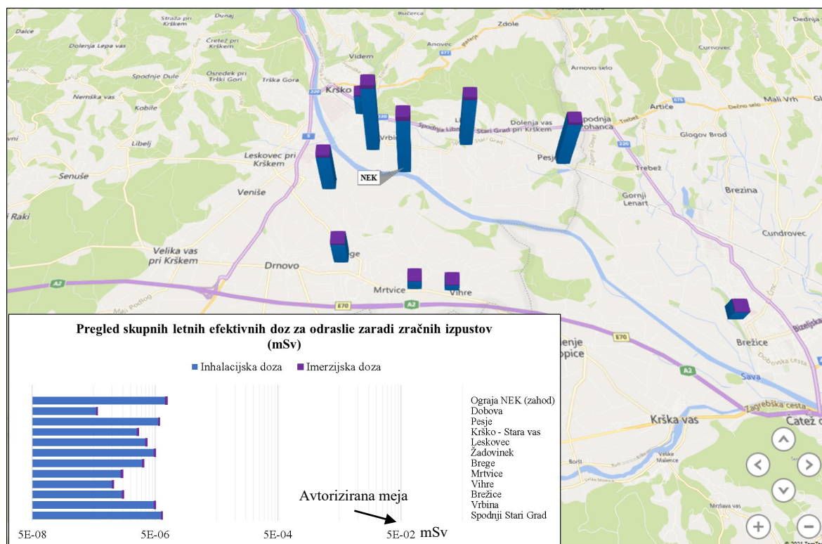
Slika P3: Pregled ocenjenih letnih efektivnih doz za umetne radionuklide za zračne izpuste v okolici NEK v letu 2020
