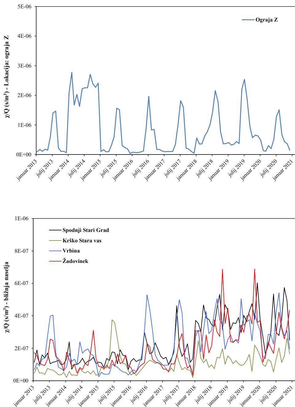
Slika 4.6: Povprečni mesečni razredčitveni koeficienti ( \chi/Q ) z enoto \text{s/m}^3 , izračunani po Lagrangeevem modelu za izpust z višine 60 m za okolico NEK za leta 2013–2020. Podatke je izračunal in posredoval MEIS, storitve za okolje.
