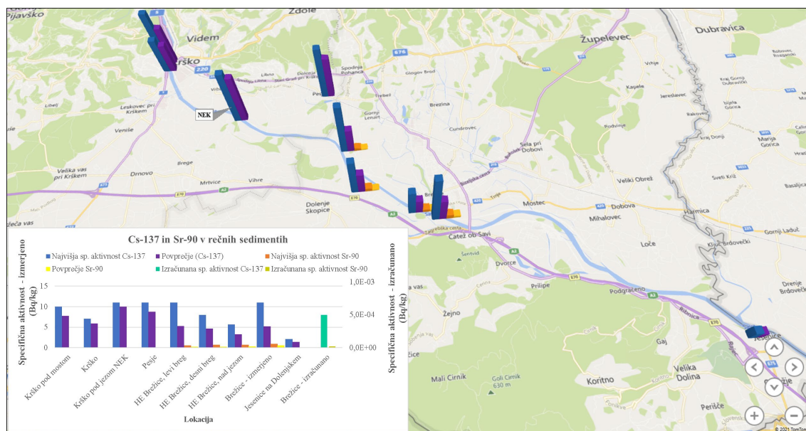
Slika I3: Specifične aktivnosti Cs-137 in Sr-90 v sedimentih v letu 2020
