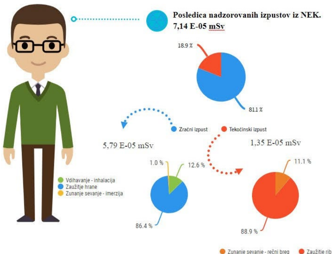
Slika P1: pregled ocenjenih letnih efektivnih doz za umetne radionuklide v okviru nadzora radioaktivnosti v okolju v okolici NEK v letu 2020
