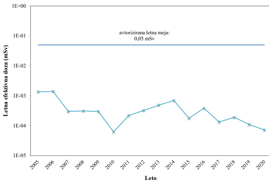
Slika I15: Seštevek ocenjenih letnih efektivnih doz posameznih referenčnih skupin zaradi emisij NEK od leta 2004 do leta 2020. Označena je tudi avtorizirana letna meja (0,05 mSv).
